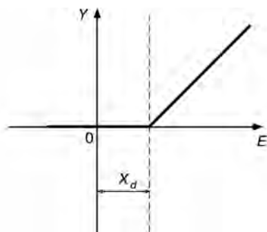
Рис. 3.12. Зона нечувствительности для исполнительного устройства типа "нагреватель"
