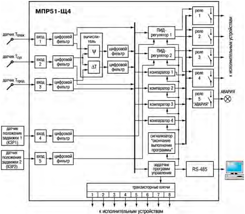
Рисунок 3.1. Структурная схема
