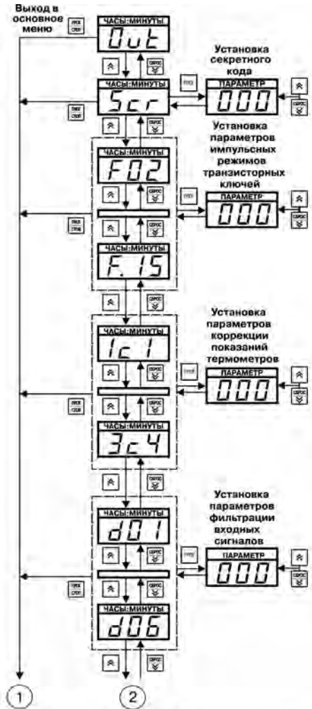
Рис. 4.3. Схема, поясняющая программирование на уровне L2
