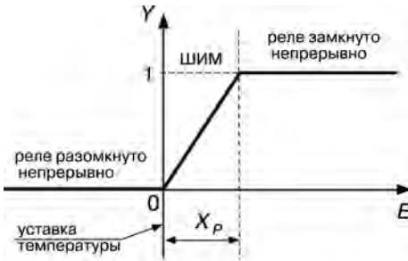
Рис. 3.7. П-закон регулирования
